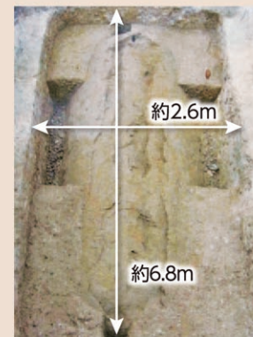
長尾山古墳粘土槨
